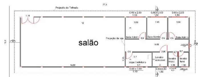
PROJETO BASICO
