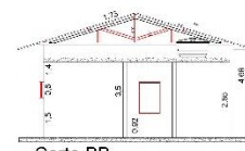
Corte BB
