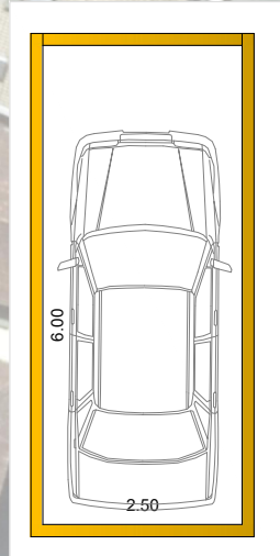
Detalhe vaga de veículos em 90°
