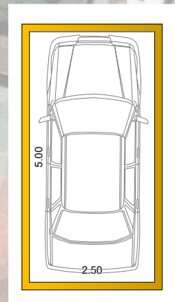
Detalhe vaga de veículos em 45°
