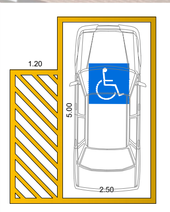
Detalhe vaga acessível
